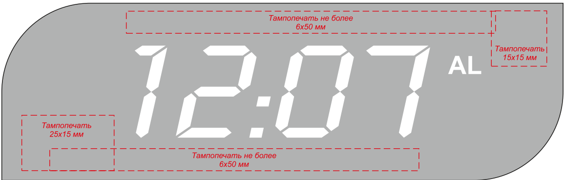
Вид спереди
