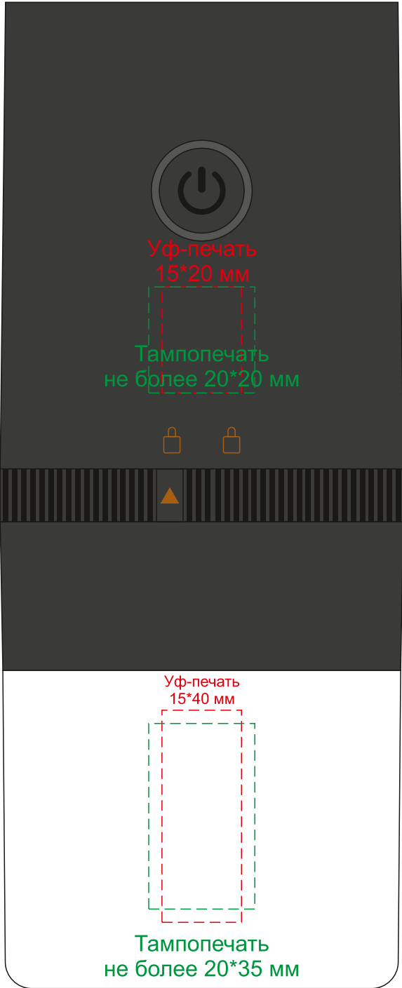
вид спереди
