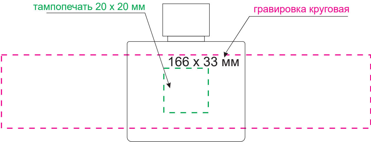
Диффузор
