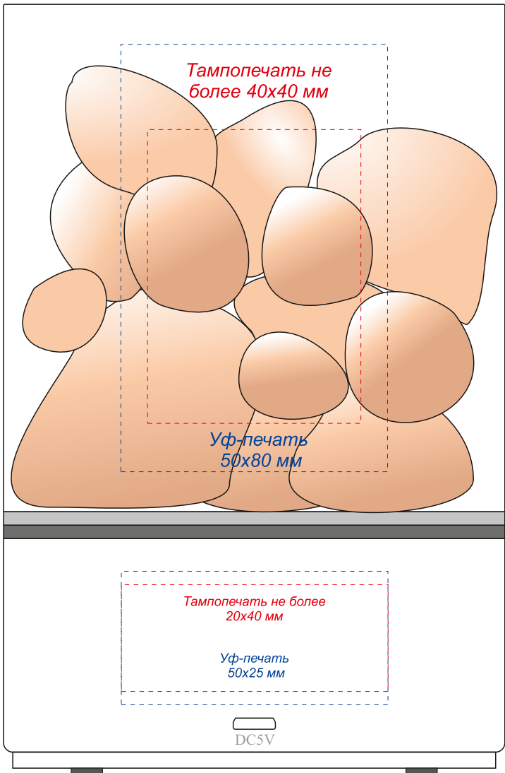
вид сзади
